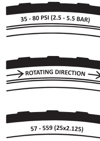
Рис. 11: Информационные надписи на боковинах покрышек
