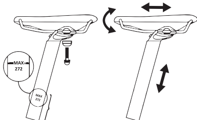
Рис. 3.1: Метка минимального углубления подседельного штыря
