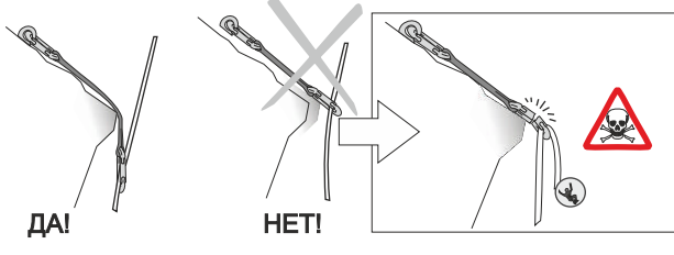
Рис. 6. Использование оттяжек с рапидами «Link 8»
