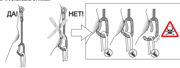
Рис. 4. Установка оттяжек
