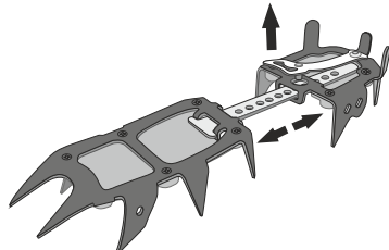
Рис. 3. Регулировка длины кошек
