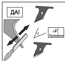
Рис. 6. Проверка и заточка зубьев
