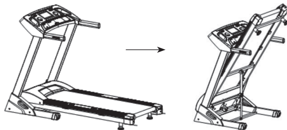
Складывание беговой дорожки
