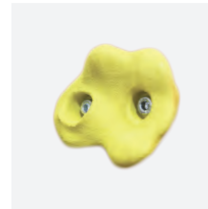
Рис. 1 – Крепление зацепа (на рис. 1) осуществляется с помощью винта с внутренним шестигранником m8*25 и крепится в оба гнезда зацепа.
